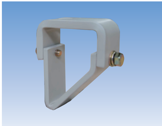
■ 山形補強金物A ● 六角ボルト M8×22 SW1、FW1付 132401 (山形鋼 50×50×6用) 132404 (山形鋼 65×65×6用)
