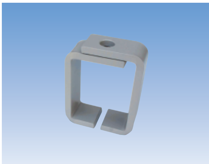
■ リップ溝形補強吊金物 132501 (リップ溝形鋼 75×45×15×2.3用) 132502 (リップ溝形鋼 100×50×20×3.2用) 132503 (リップ溝形鋼 120×40×20×3.2用)
