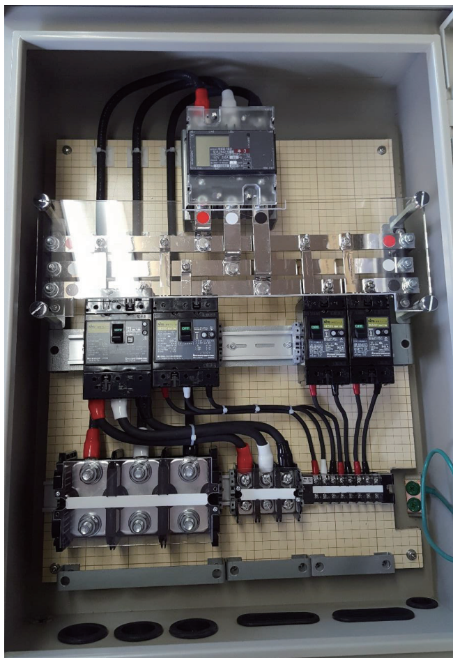
交流分電盤
