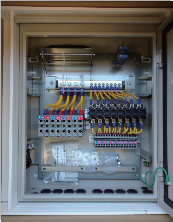
(光8芯電源8分岐盤)
