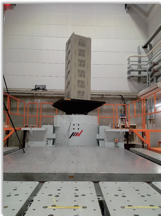
3G(X/Y/Z軸)加振による強度試験クリア
