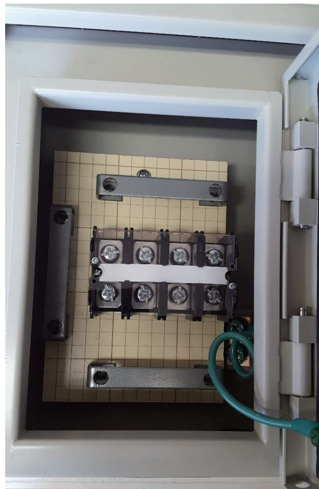
直流中継盤
